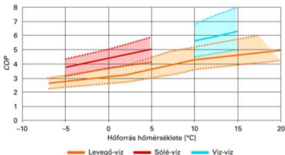
2. ábra. COP [kW/kW] mérési eredmények (a hőszivattyú teljesítménytényezője 35 °C előremenő vízhőmérséklet esetén)
